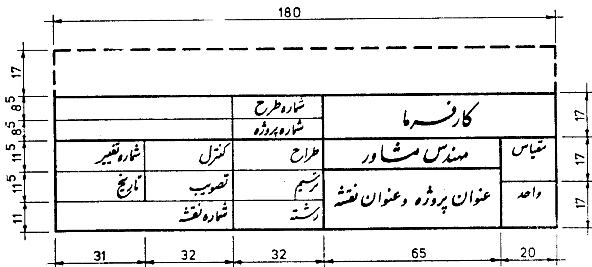
جدول ۲- اندازه جدول عنوان نقشه برای کاغذ A ۴
