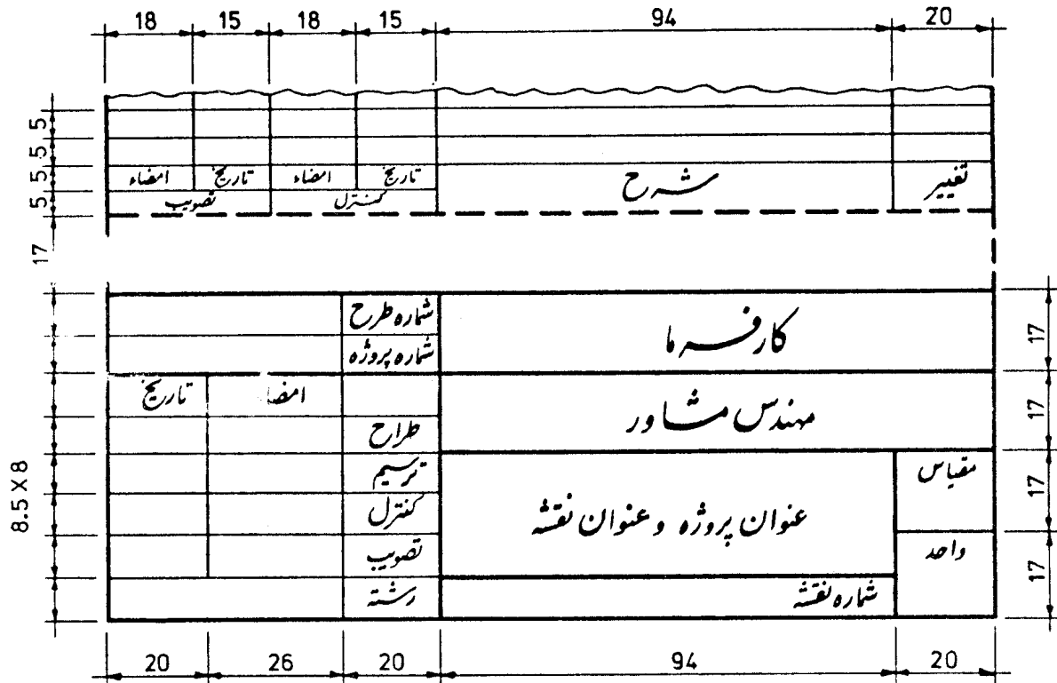
جدول ۱- اندازه جدول عنوان نقشه برای کاغذهای استاندارد A ۰ , A ۱ , A ۲ و A ۳
