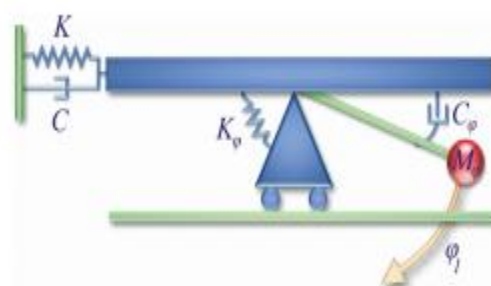
شکل 2-4: مدل گسسته S-R برای یک پی سطحی
