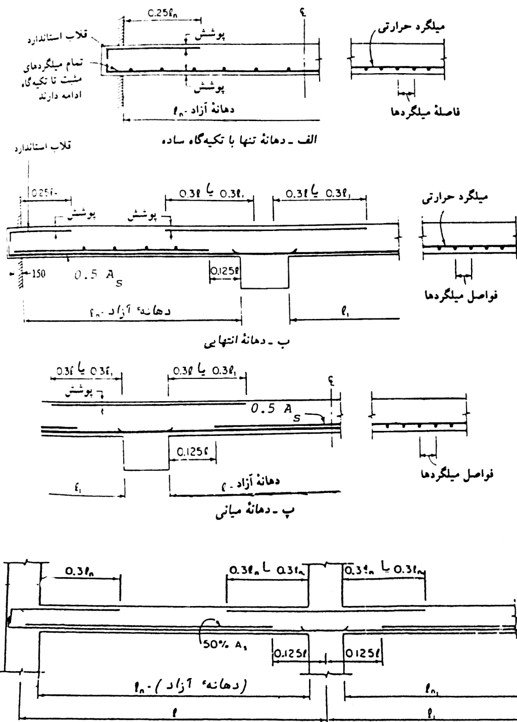
شکل ۱۰-۱۴ - نقاط تسليع میلگردها در دالهای دو طرفه
