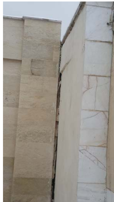
شکل ۱۶- عدم پوشش مناسب درز انقطاع و چسبیدن آن به ساختمان مجاور بوسیله مصالح سنگی نما و پرکردن این فاصله با خرده سفال
