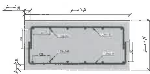
برش A-A
