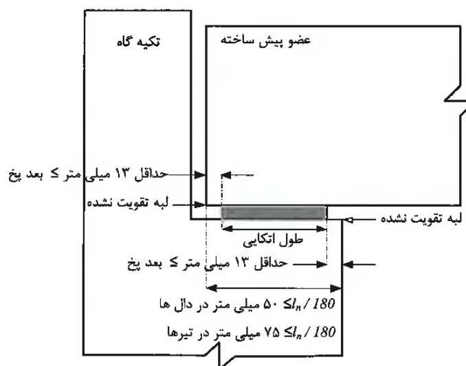
شکل ۵-۱۷-۹ حداقل ابعاد در اتصالات اتکایی
