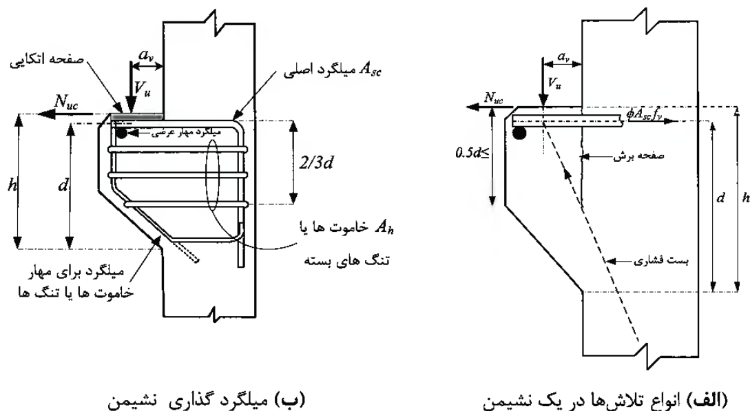
شکل ۱-۱۷-۹ نمایش یک نشیمن و نیروهای وارد بر آن
