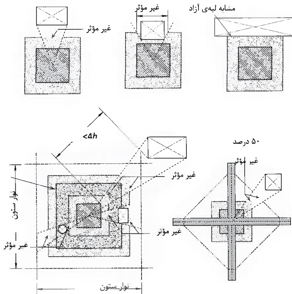
شکل ۸-۹-۱ تأثیر بازشو در دال بر سطح مؤثر مقطع بحرانی
