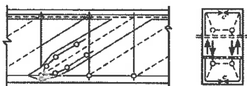
پ- عضو فشاری قطری در جابجایی خالص
