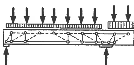
الف- تیر و کنسول با تکیه گاه ساده
