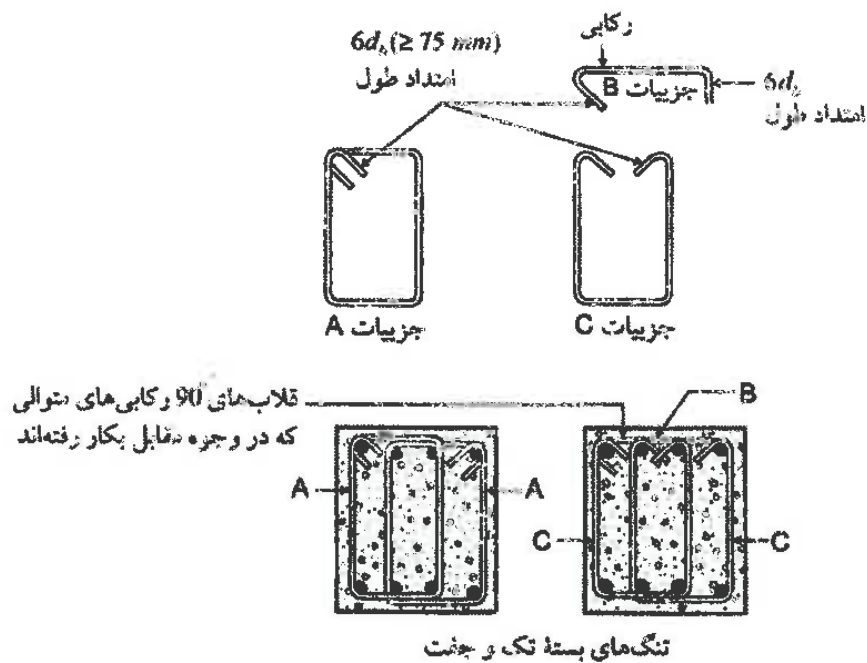
شکل ۹-۶ پ-۴ جزئیات اجرایی دورگیرها
